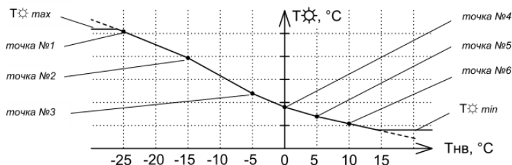
Рисунок 11 – Температурный график
