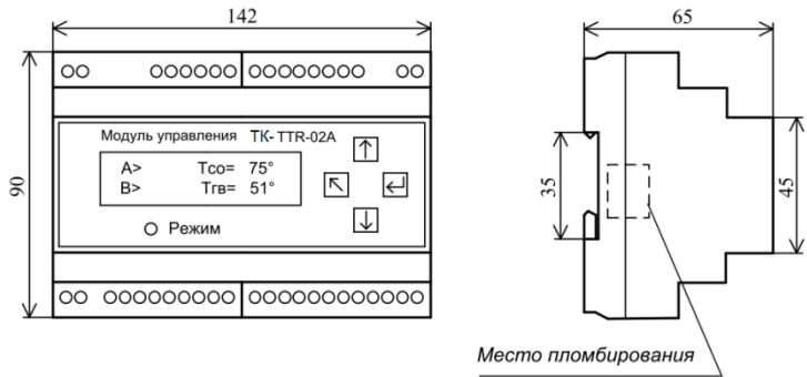
Рисунок Б.1 - Общий вид и габаритные размеры
