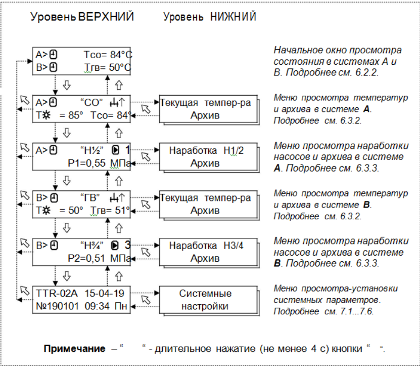
Рисунок 3 – Общая структура пользовательского меню
