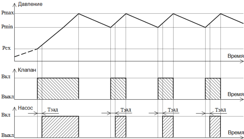
Рисунок 2 – Диаграмма работы по управлению подпиткой
